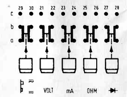
Miniatürkstenschalter (Bestückungsseite) MINIATURE KEY-SWITCH (COMPONENT SIDE) 40102-032.00
